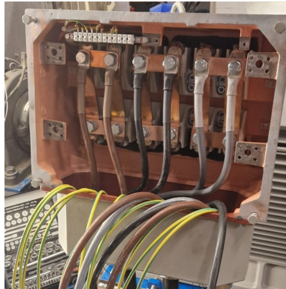
Demontage Anschluss bestehenden Motor 500kW
